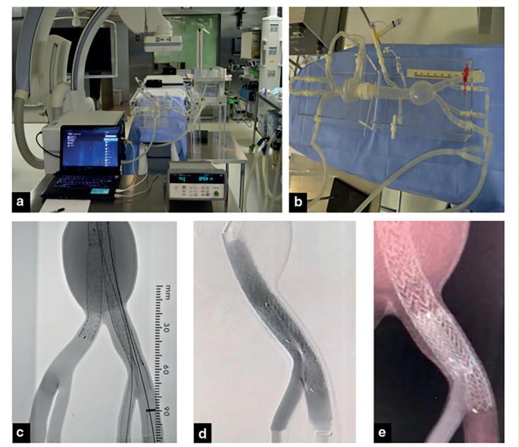
Fig 3 - a. e b. Modelo de aneurisma e sistema de fluxo na sala de avaliação; c. Fluoroscopia; d. Angiografia; e. Avaliação durante o teste in-vitro.
